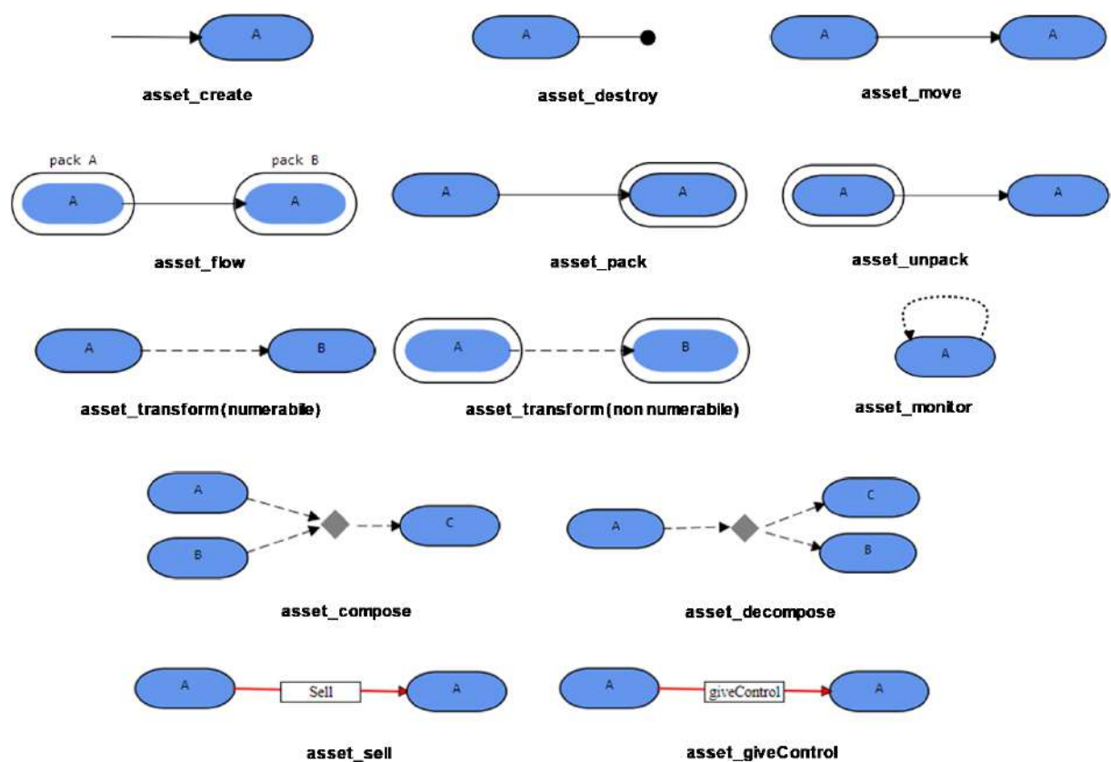
Figura 11. Operazione del nostro modello.
